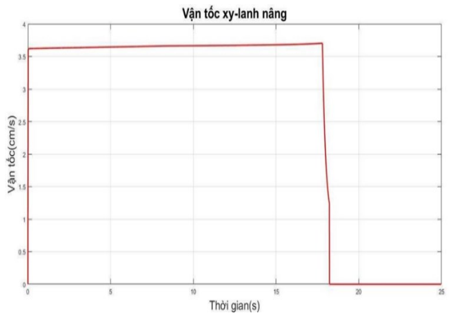
Hình 19. Đồ thị vận tốc xylanh nâng giai đoạn 2 – nâng thùng đầy tải
