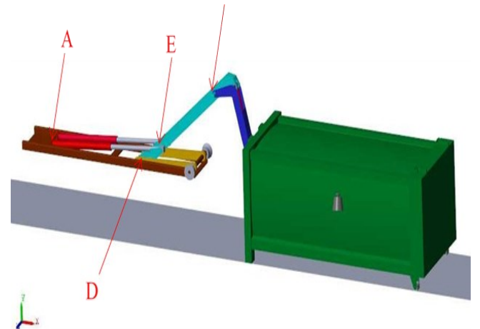
Hình 9. Mô hình mô phỏng và vị trí các chốt ở giai đoạn 1 khi nâng thùng đầy tải
