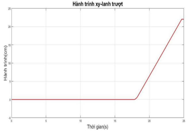
Hình 18. Đồ thị hành trình xylanh trượt giai đoạn 2 – nâng thùng đầy tải
