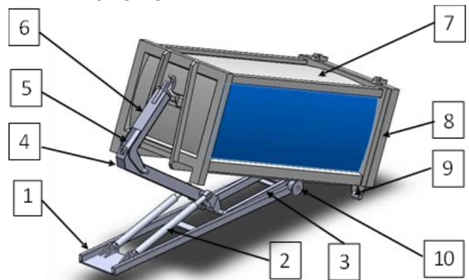
Hình 1. Cấu tạo bộ công tác nâng hạ thùng rời 1: Khung phụ, 2: xy-lanh nâng, 3: Tay khuỷu, 4: Tay nâng, 5: Xy-lanh tay quay, 6: Tay quay, 7: Thùng chứa, 8: Nắp thùng chứa, 9: Bánh xe thùng chứa, 10: Bánh lăn.
