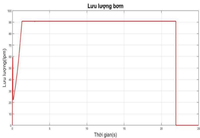
Hình 13. Đồ thị lưu lượng bơm ở giai đoạn 1 – nâng thùng đầy tải có thời gian
